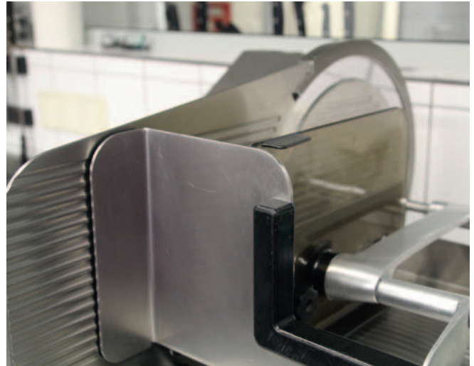
Abb. 7 Sicherheitseinrichtungen an der Aufschnittschneidemaschine; Fingerschutz am Schlitten, Restehalter und Messerschuttring
