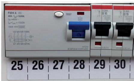
Abb. 4: Fest eingebauter RCD (links) und Leitungsschutzschalter (rechts)
