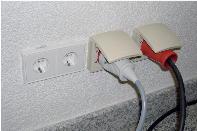
Abb. 2: Vollständige Isolierung von Kabeln, Steckern und Steckdosen
